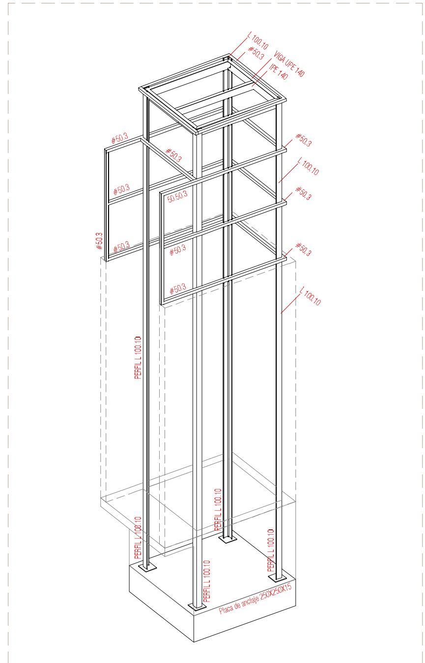
AXONOMETRÍA ESTRUCTURA ASCENSOR
