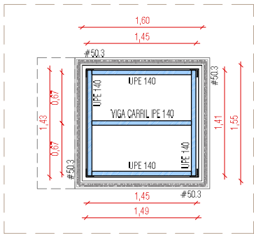
PLANTA CUBIERTA E:1/50
