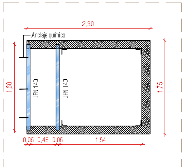
SUELO PLANTA PRIMERA E:1/50
