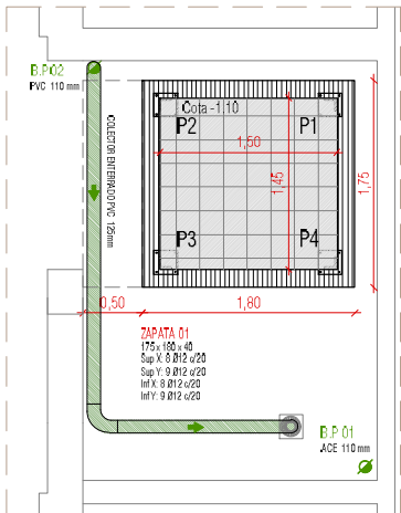
PLANTA CIMENTACIÓN E:1/50
