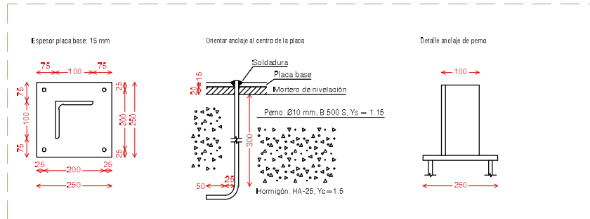
DETALLE PLACA DE ANCLAJE E:1/10
