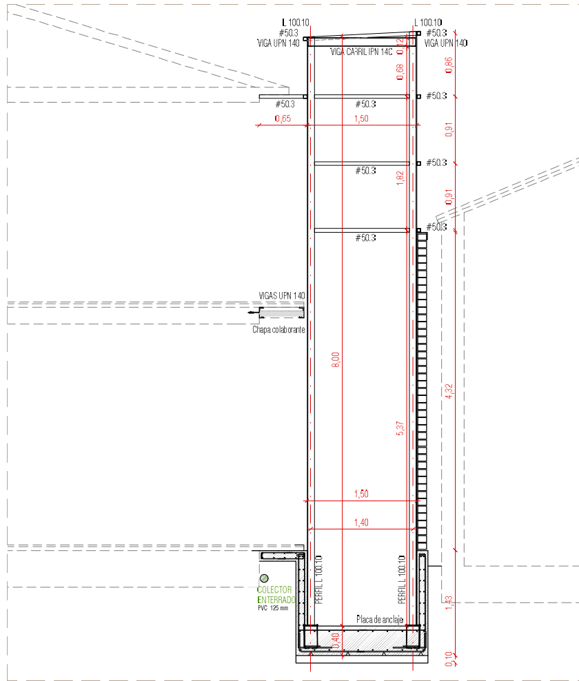
SECCIÓN ESTRUCTURA ASCENSOR E:1/50
